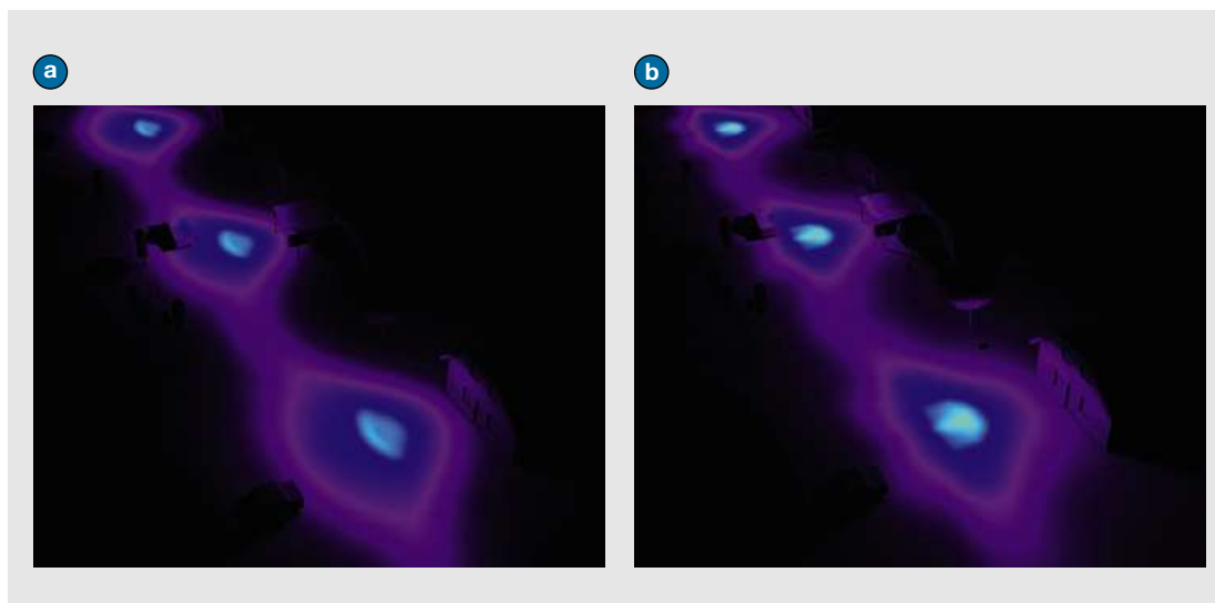
Bild 2 Lichtverteilung von a) LED (37 W pro Leuchte) und b) Natriumdampf (60 W pro Leuchte) bei einer Quartierstrasse.
