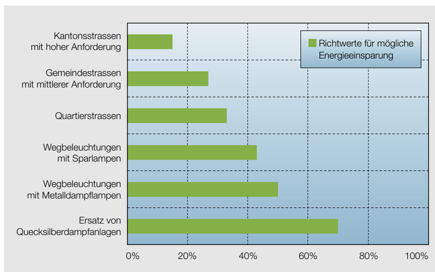
Bild 3 Energiesparpotenzial aus EKZ-Erfahrungen bei Neuanlagen und bestehenden Anlagen mit idealen baulichen Gegebenheiten und den derzeit besten LED-Leuchten.
