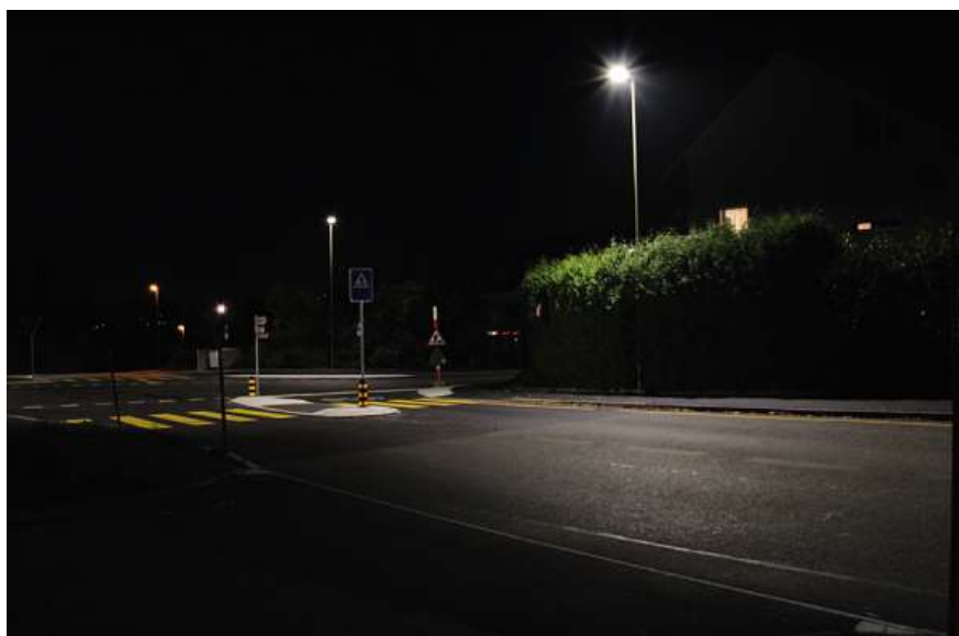
Bild 4 Dank der Richtwirkung ermöglicht die LED-Beleuchtung eine helle Strasse bei dunkler Fassade.
