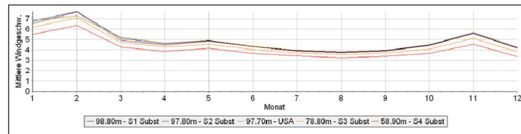
Abbildung 38: Jahresgang der mittleren Windgeschwindigkeit (Auswertungsperiode).
